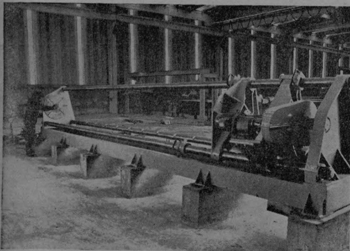
Esta fotografía muestra la máquina especial para cortar, a determinados tamaños, los tubos de asbesto-cemento que a partir del próximo mes de enero, estará fabricando RICALIT, S.A., en su nueva fábrica de tubos instalada en Paraíso de Cartago.
